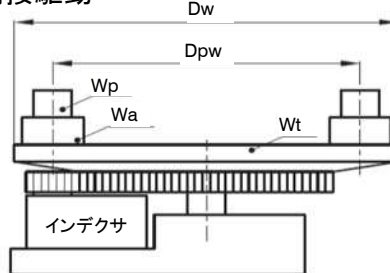
間接駆動
