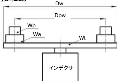
直接駆動
